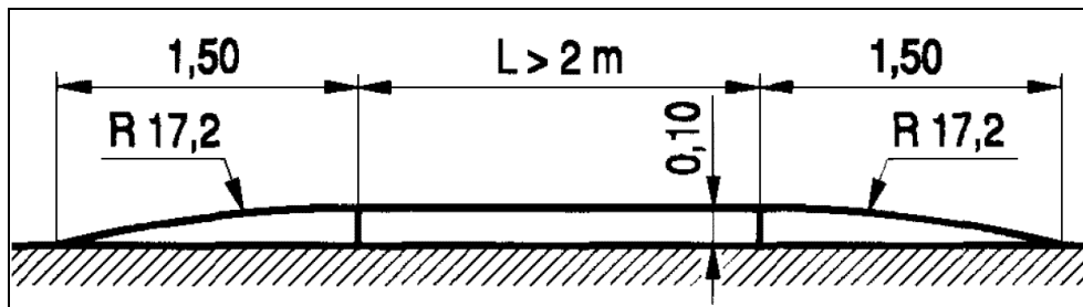
3.2. Próg płytowy z powierzchniami najazdowymi łukowymi (U-16b)
