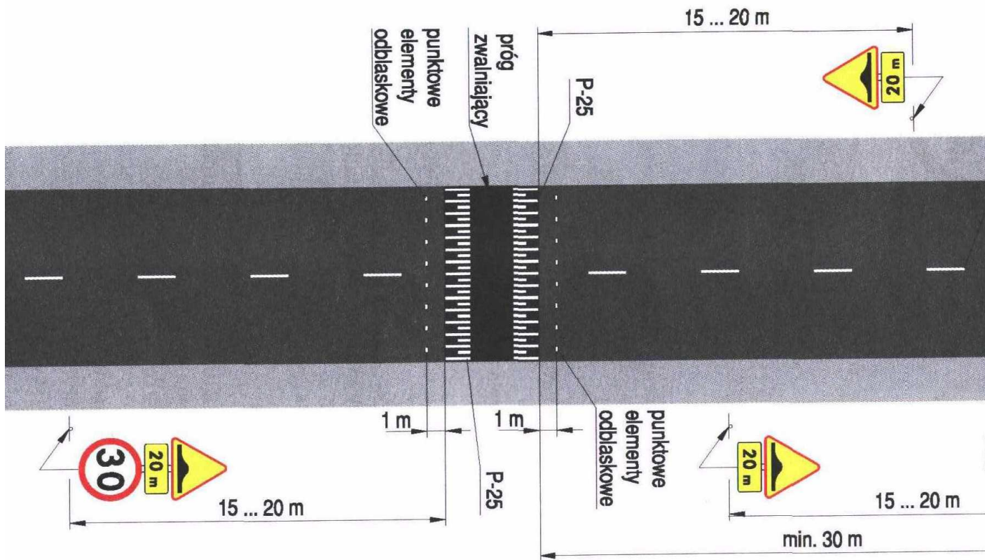
Rys. 3. Przykład oznakowania pionowego i poziomego odcinka drogi, na którym znajdują się dwa progi zwalniające U-16c i próg płytowy z wyniesionym przejściem dla pieszych
