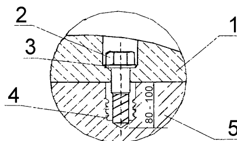
Szczegół A
